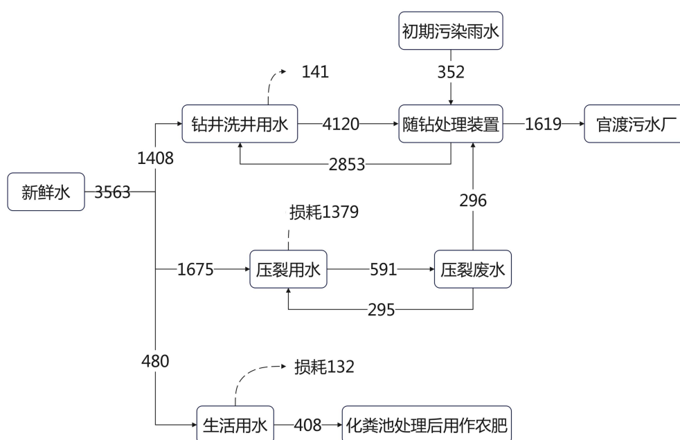
图2-7 本项目水平衡图（单位：t）
