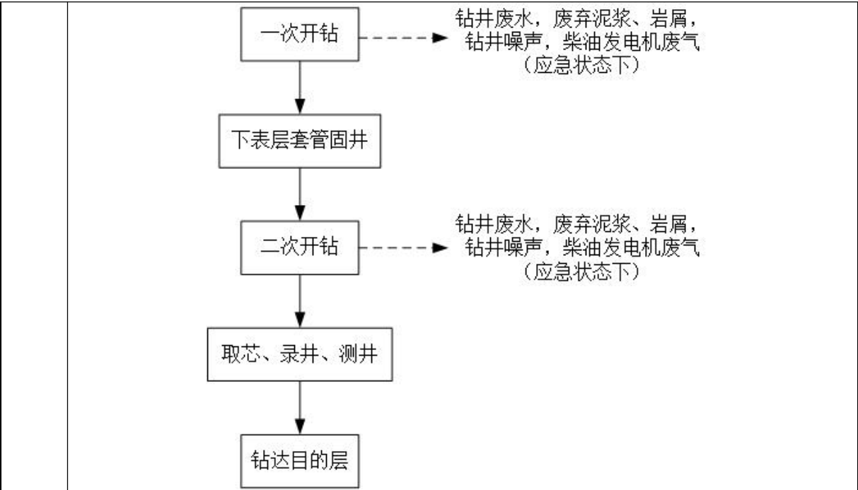
图2-5 钻井工艺流程图
