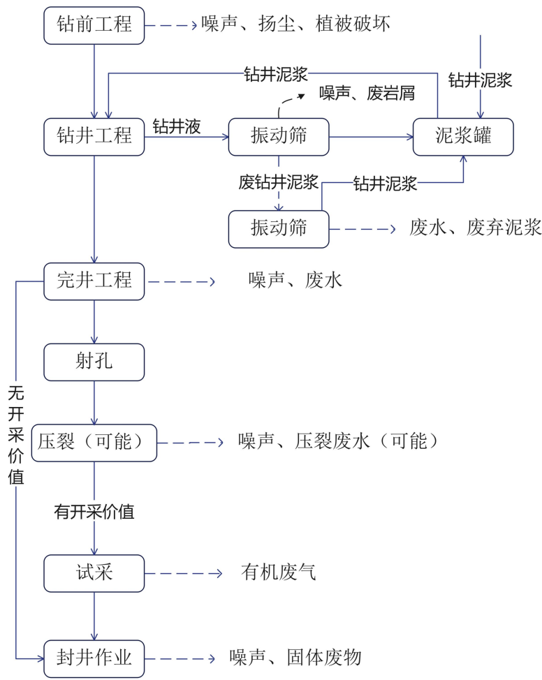
图2-4 施工工艺流程及产污环节图
